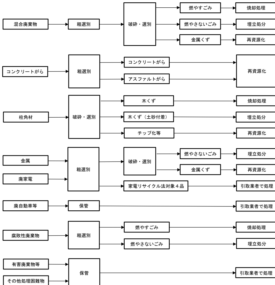
図10 処理基本フロー
