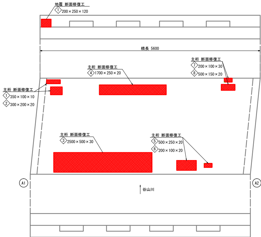
平面図（桁下） S=1:30
