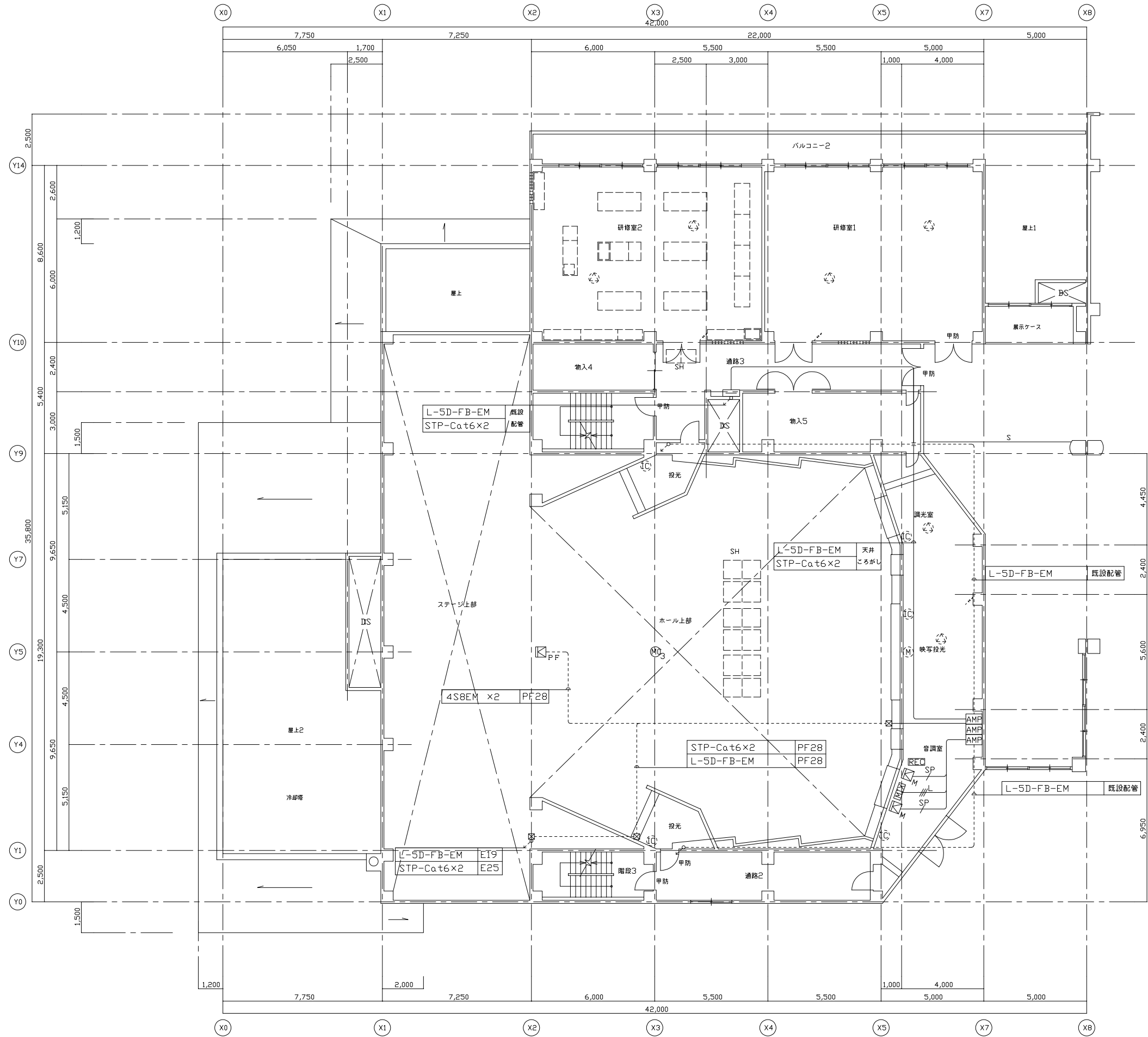
3階平面図
