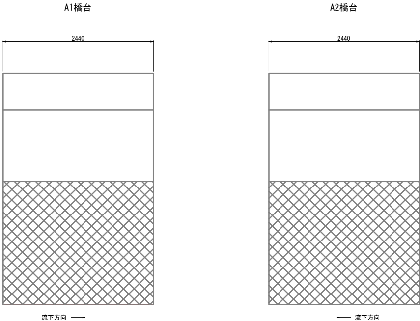
下部工断面図 S=1:30
