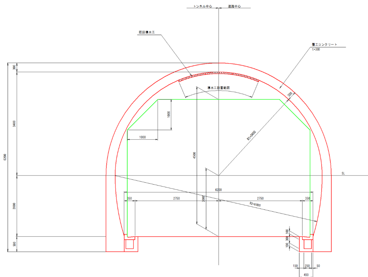
【奥山田隧道標準断面図】
