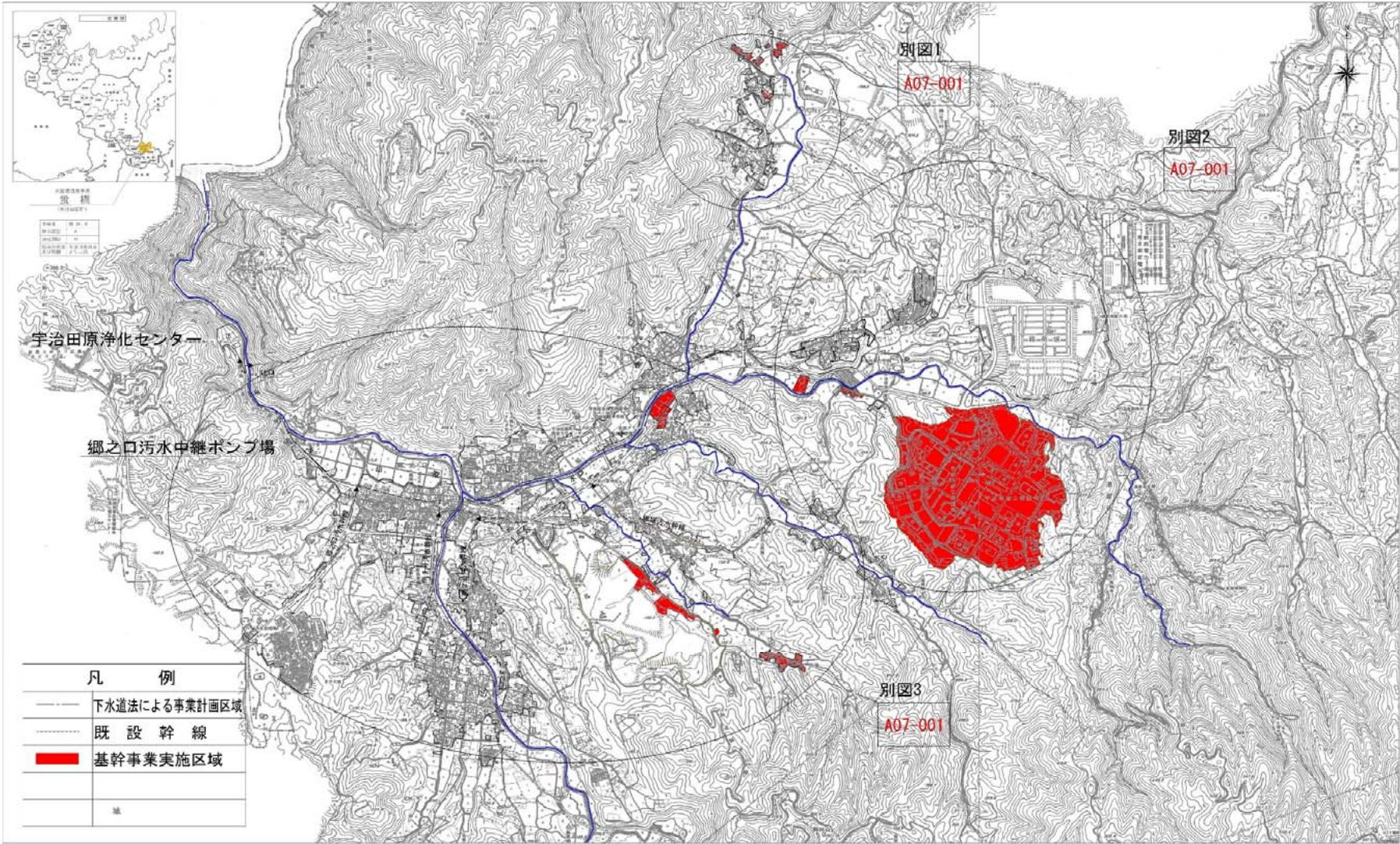
宇治田原町公共下水道計画図（污水）
